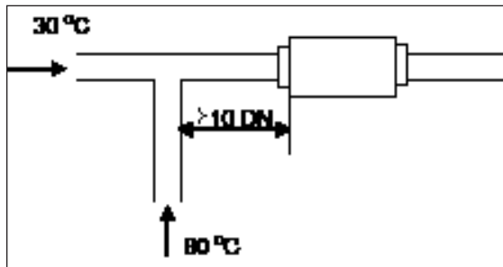
Mischung unterschiedlicher Rücklaufemperaturen
