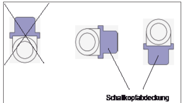
Zulässige Einbaulage bei Kältezählung
